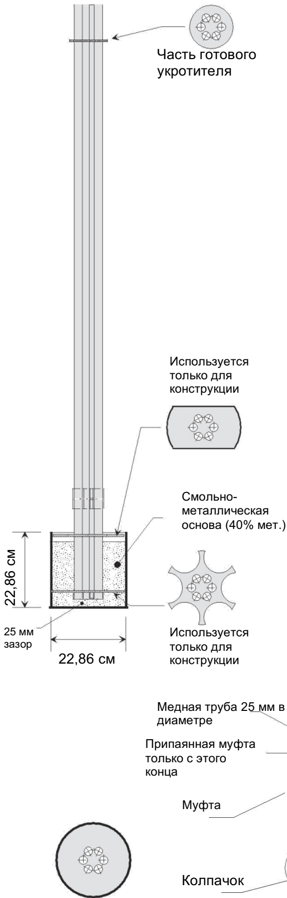
СХЕМА
